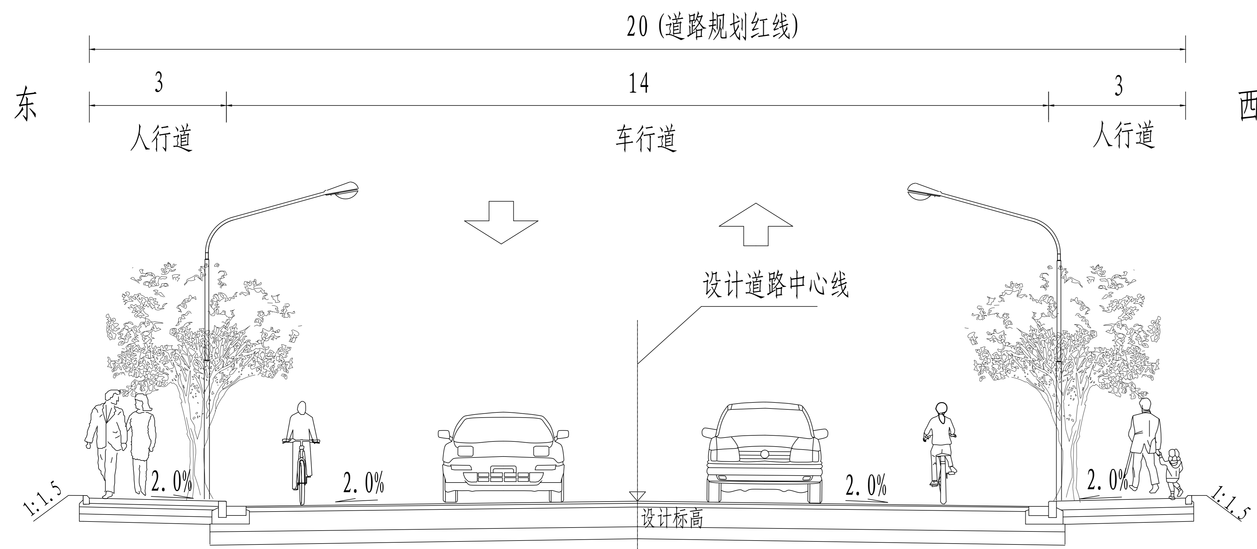
道路标准横断面图
