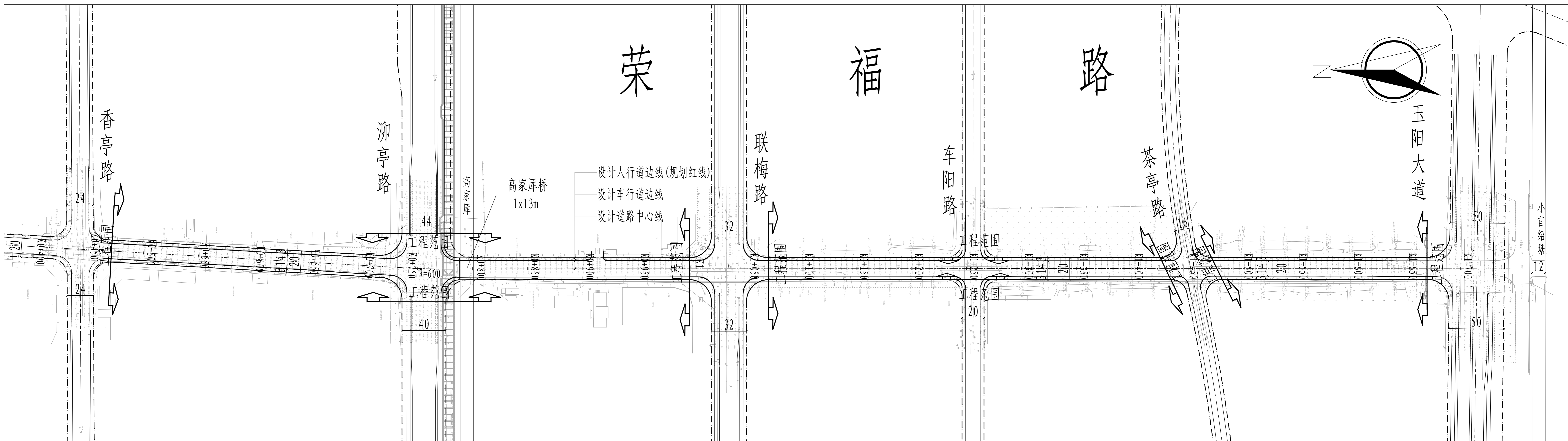
荣福路(香亭路-玉阳大道)平面设计图
